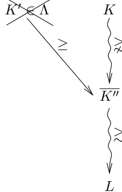
(d) K strongly covers L in \Lambda .
